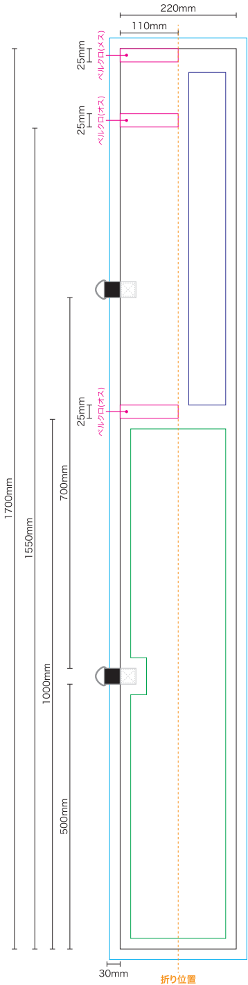
展開図
