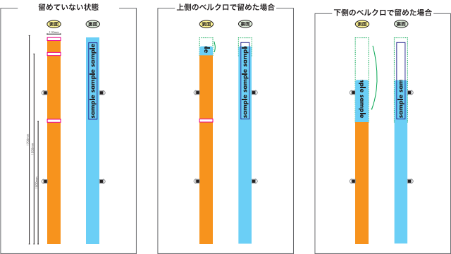
展開図
